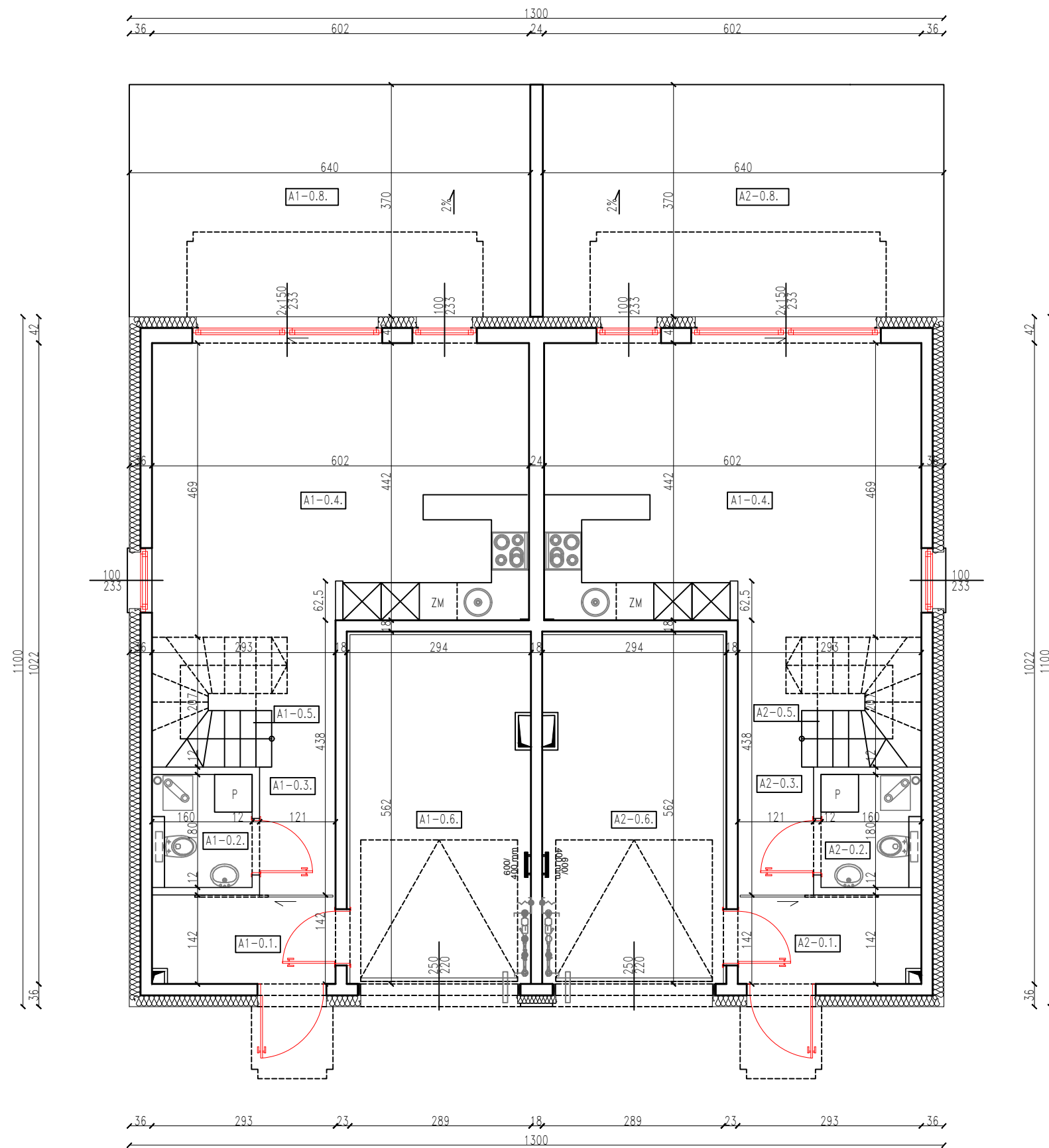
RZUT PARTERU
